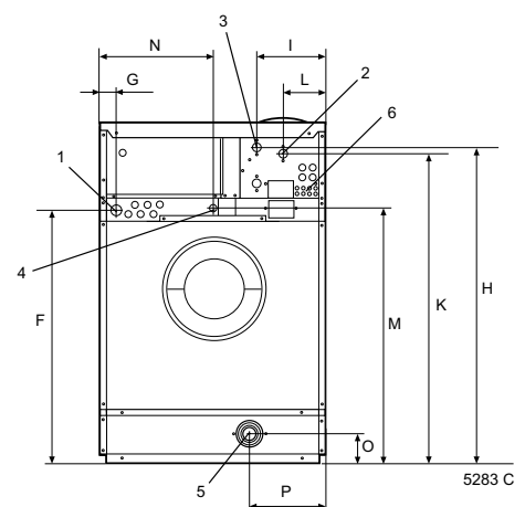
Achterzijde
