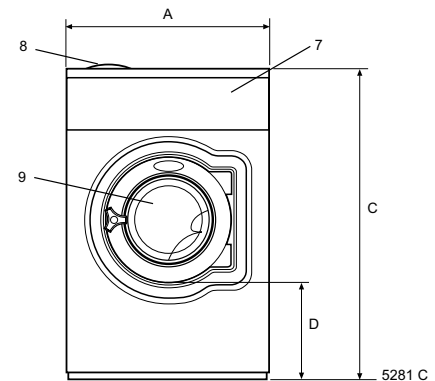
Voorzijde
